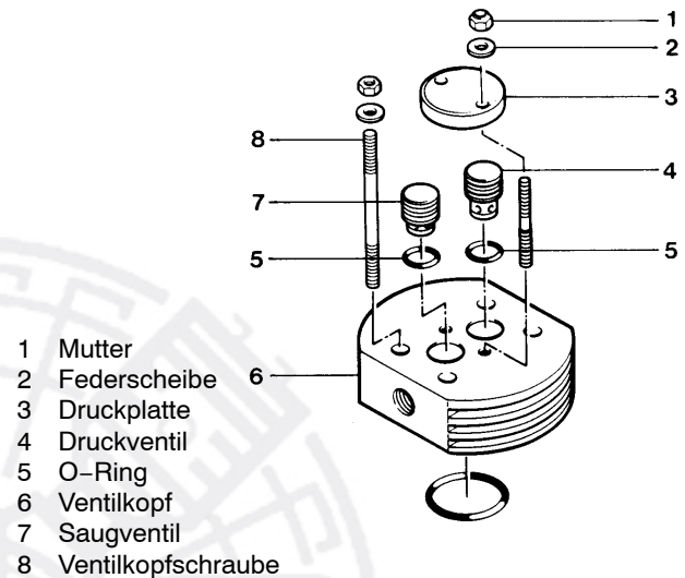
Abb. 37 Ventilkopf 2. Stufe
