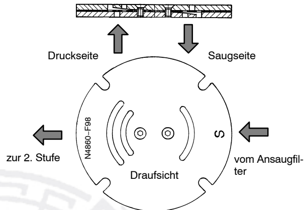
Abb. 35 Ventil 1. Stufe
