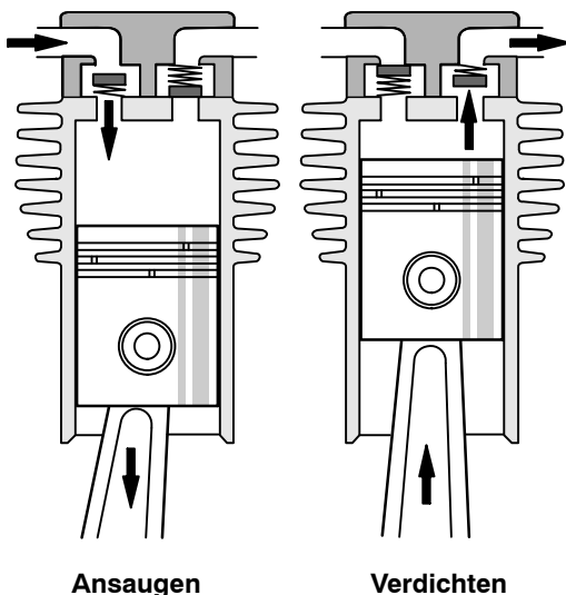
Abb. 34 Ventil-Arbeitsweise
