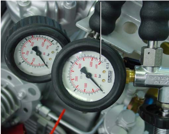
Abb. 33 Enddruckmanometer
