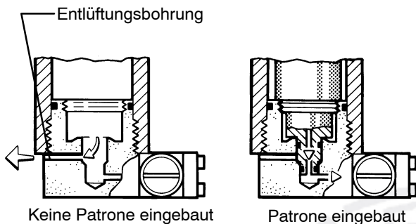
Abb. 30 Entlüftungsbohrung
