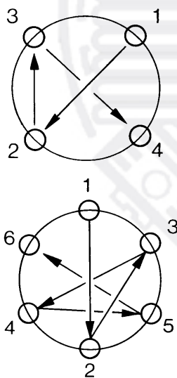
Abb. 44 Anzugsreihenfolge
