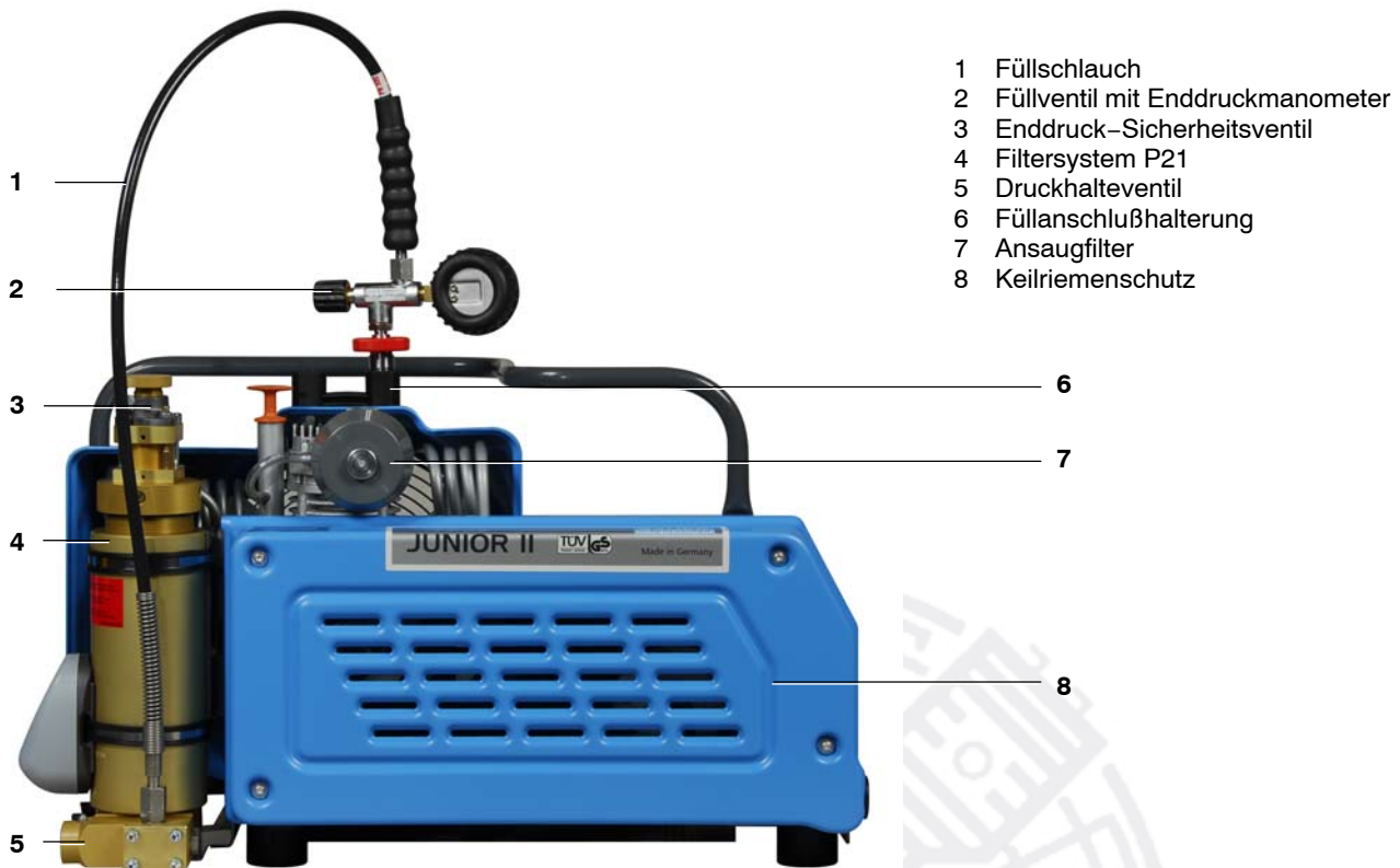
Abb. 4 Kompressoranlage mit Elektromotor , Schwungradseite
