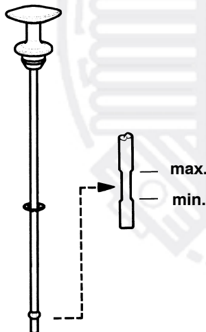
Abb. 26 Ölpeilstab-Markierungen
