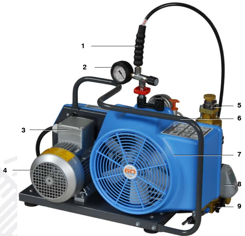
Abb. 2 Kompressoranlage mit Elektromotor (Drehstromausführung)
