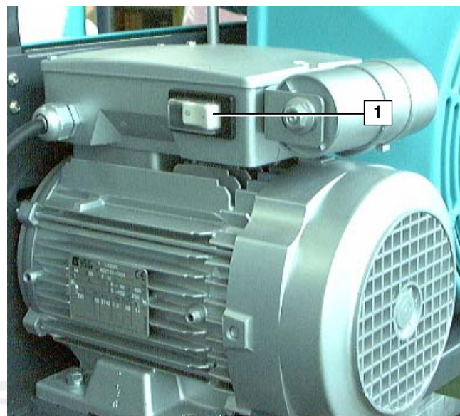
Abb. 42 Motorschutzschalter (Wechselstrommotor)
